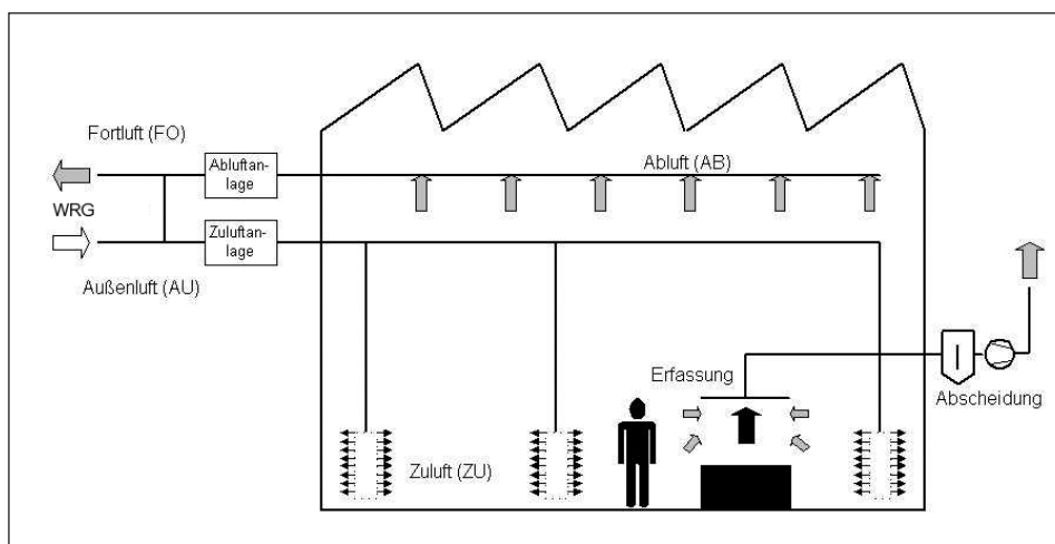
Abb. 25: Empfohlenes Lüftungskonzept mit Schichtlüftung und Fortluft
