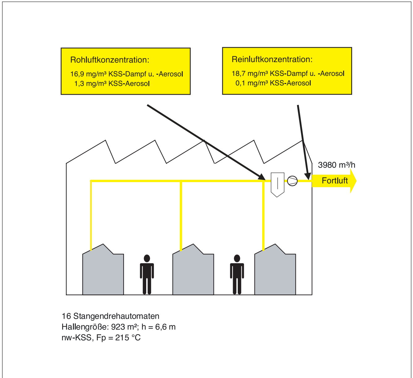
Abb. 10: Skizze zum Hallenlüftungskonzept 1, Betrieb A
