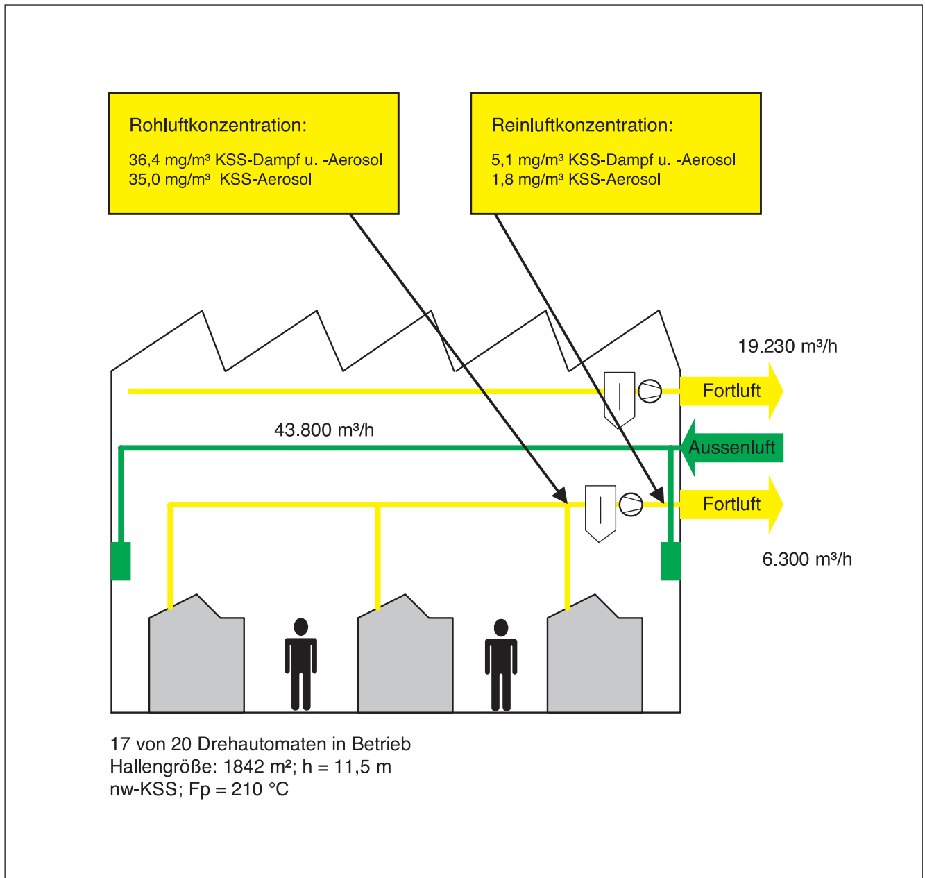
Abb. 19: Skizze zum Hallenlüftungskonzept 3, Betrieb D
