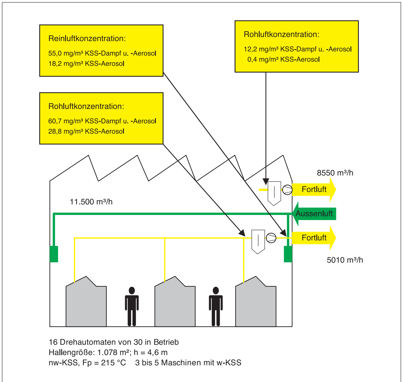
Abb. 16: Skizze zum Hallenlüftungskonzept 3, Betrieb C
