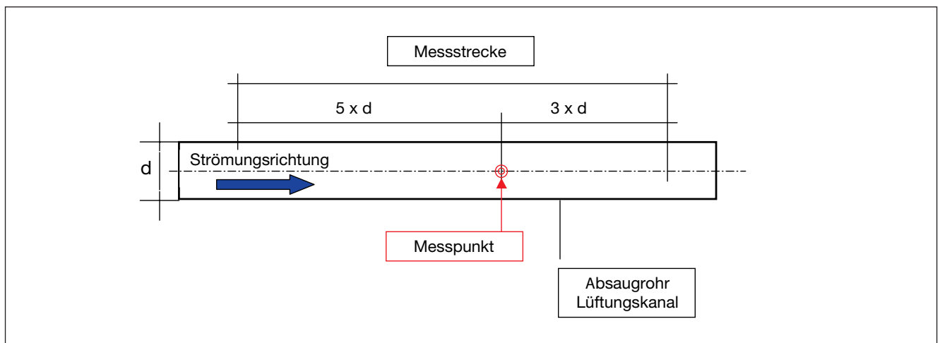
Abb. 6: Messstrecke in Rohrleitungen und Lüftungskanälen
