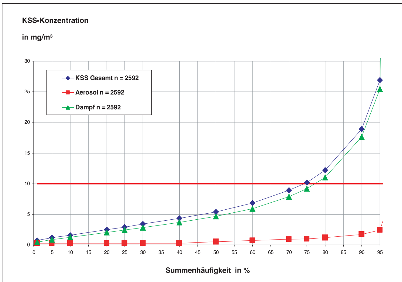
Abb. 1: Summenhäufigkeit der KSS-Konzentrationen differenziert nach KSS-Dampf und KSS-Aerosol (Quelle: BGIA)
