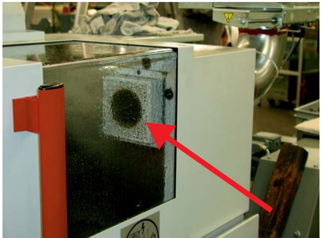
Abb. 24: Tropfenabscheider vor der Ansaugöffnung zur Minimierung des KSS-Verlustes aus der Maschine
