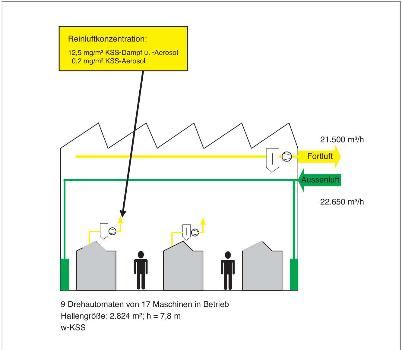
Abb. 13: Skizze zum Hallenlüftungskonzept 2, Betrieb B
