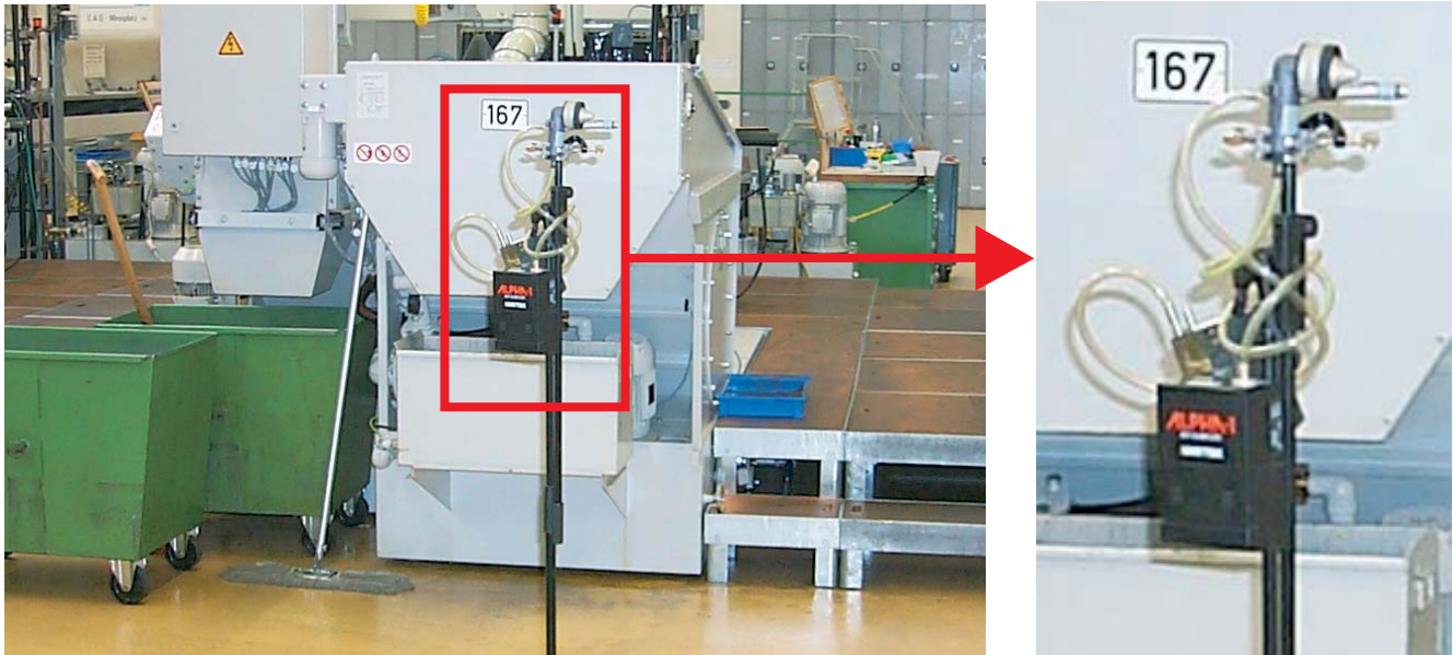
Abb. 2 und 3: Stationäre Probenahme mit PAS-Pumpe, Aktivkohleröhrchen und Gesamtstaub-Gas-Probenahmesystem (GGP), Mess- und Analyseverfahren sind detailliert in der BGIA-Arbeitsmappe „Messung von Gefahrstoffen“ unter der Kennzahl 7750 veröffentlicht.
